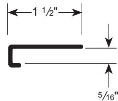
ROOF EDGE TRIM
